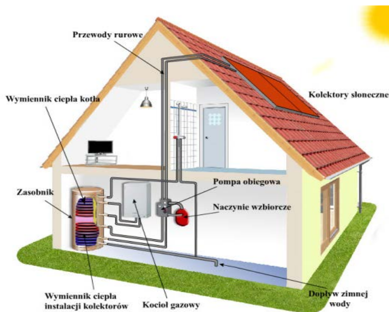
Ryc. 13. Schemat instalacji kolektorów słonecznych w domu jednorodzinnym
