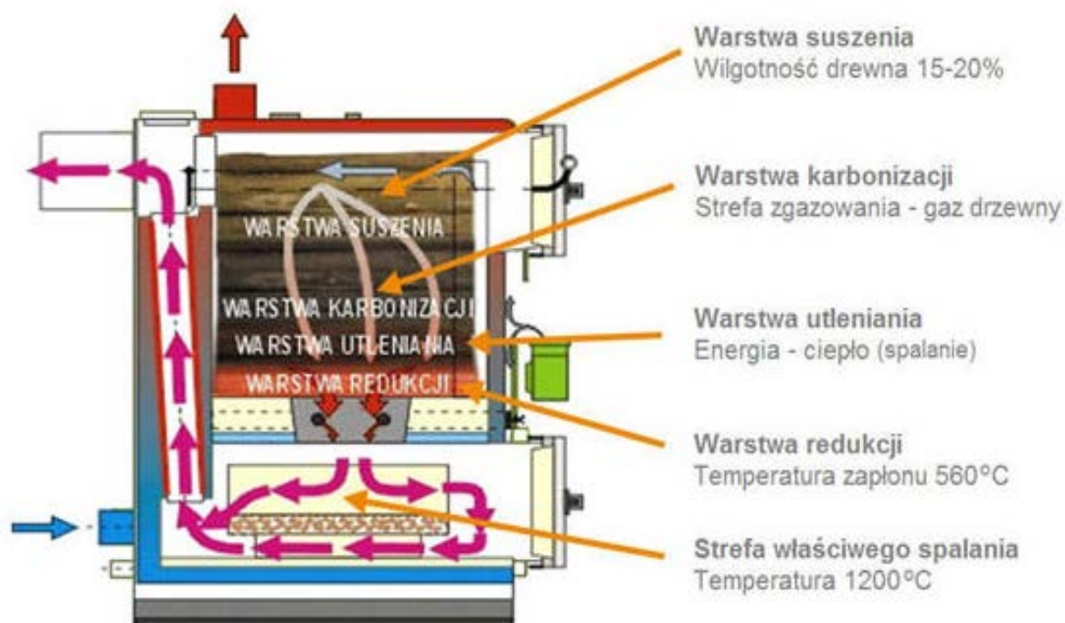
Ryc. 18. Schemat spalania drewna w kotle zgazowującym
