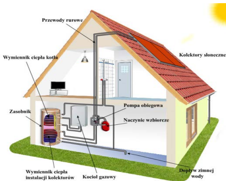
Ryc. 13. Schemat instalacji kolektorów słonecznych w domu jednorodzinnym
