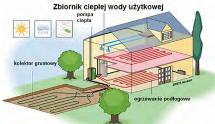
Ryc. 17. Schemat działania gruntowej pompy ciepła z kolektorem poziomym
